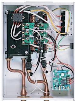
Внутренний вид котла Nobby Electro KBK
